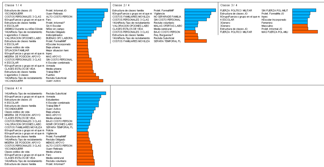
Variable: Coupure 'c' de l'arbre en 4 classes - Valeurs-test
